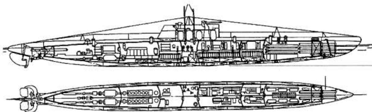
Подводная лодка типа «Д-1»
